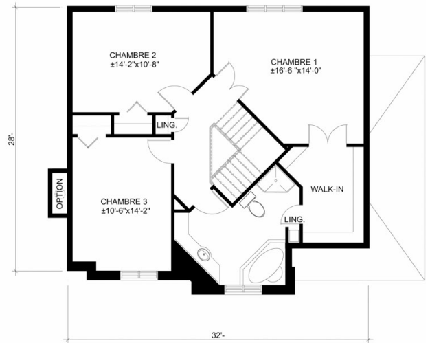
ÉTAGE 914 PL.CA
