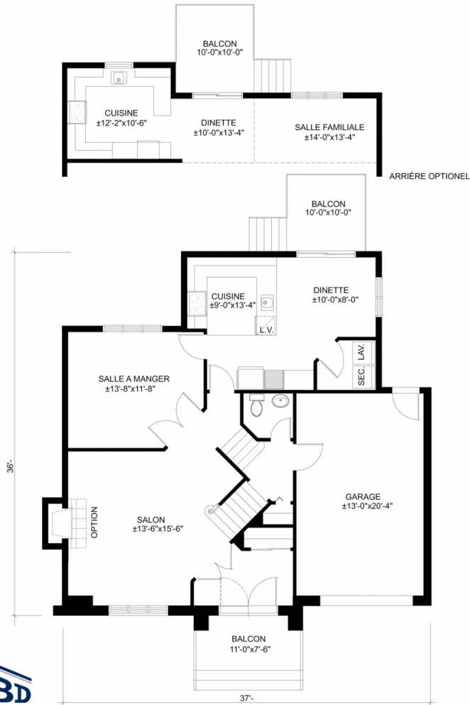
REZ-DE-CHAUSSÉE 885 PL.CA
